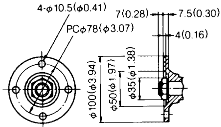
Getriebeflansch
